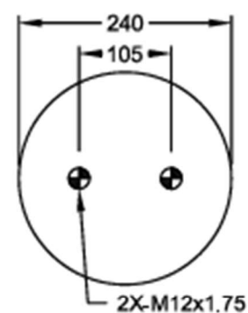
4079 PISTON
